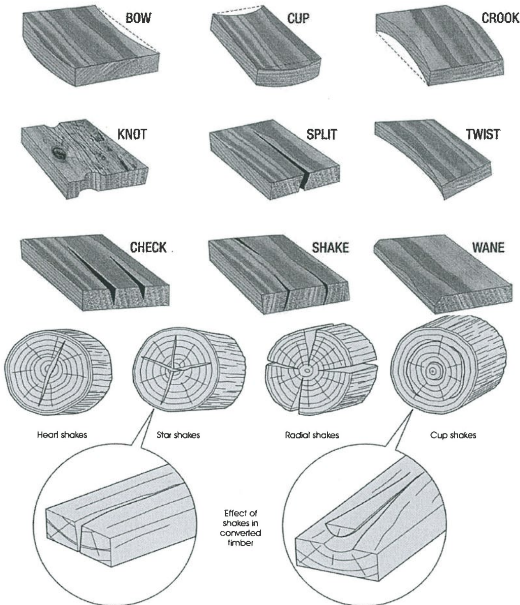
ภาพตัวอย่างลักษณะตำหนิบนไม้
